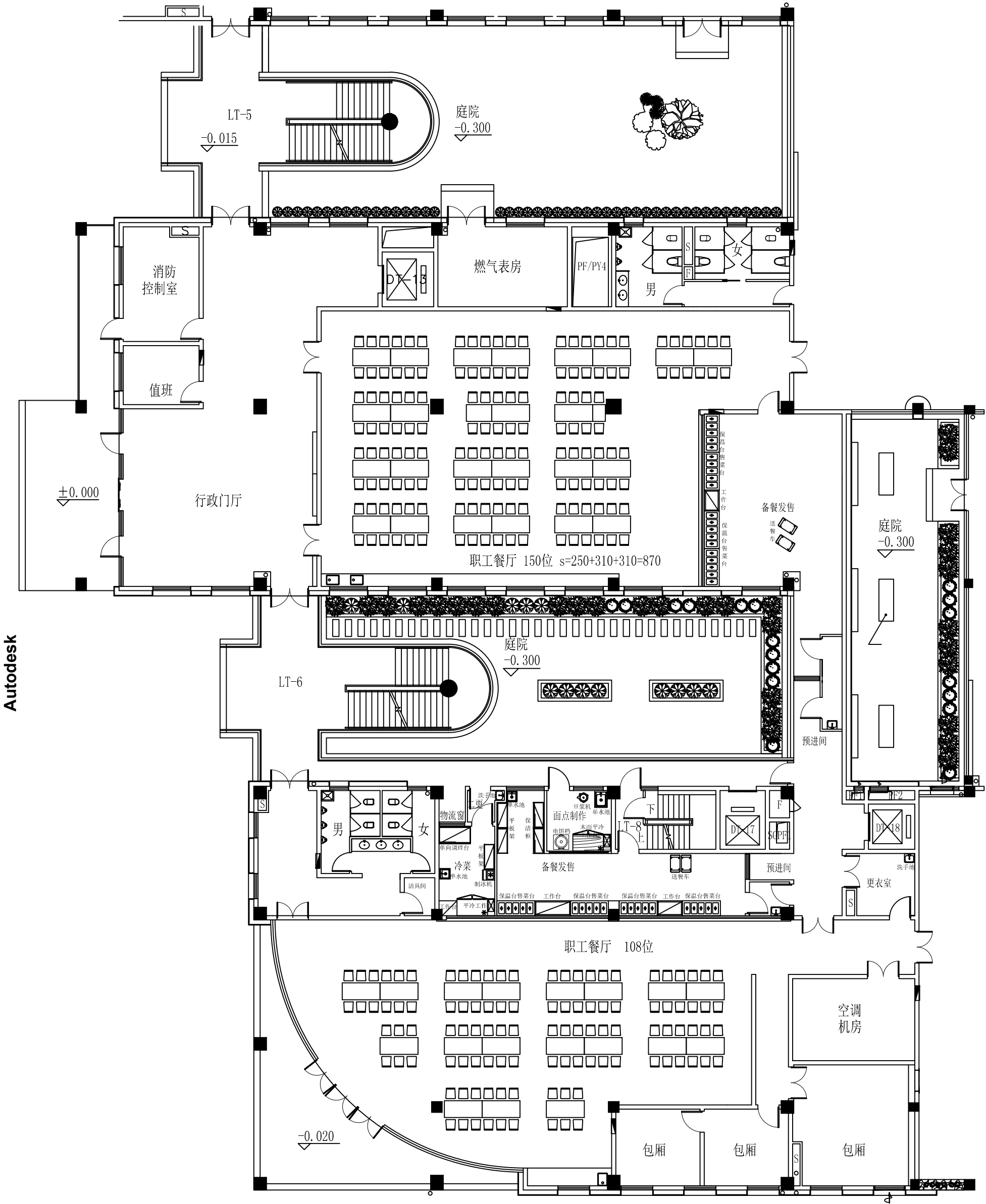
一层平面布置图
